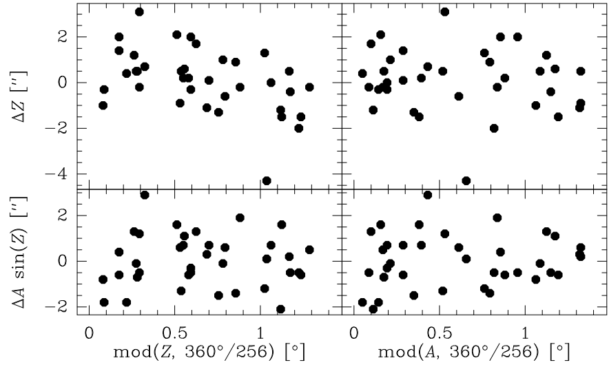
2011-03-02/2011-03-02-a.optfit.dat
